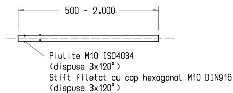
Prelungire consola semafor
