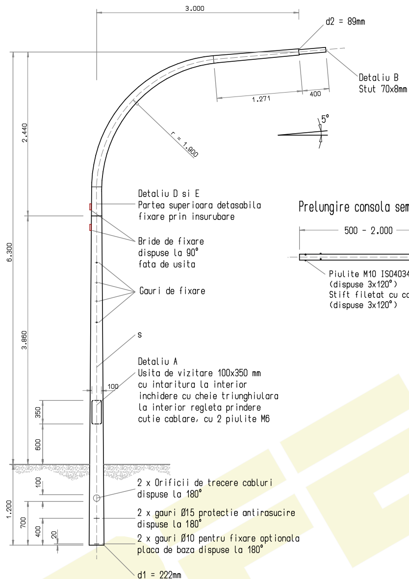
Detaliu A - Usita de vizitare
