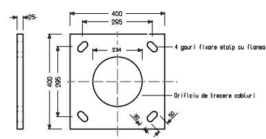
Detaliu C - Flansa de prindere
