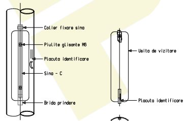
Detaliu A - Usita de vizitare
