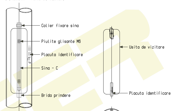
Detailu A - Usita de vizitare
