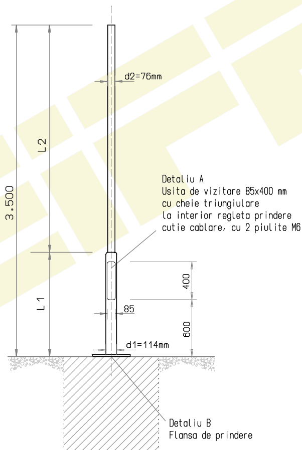
Detailu B - Flansa de prindere
