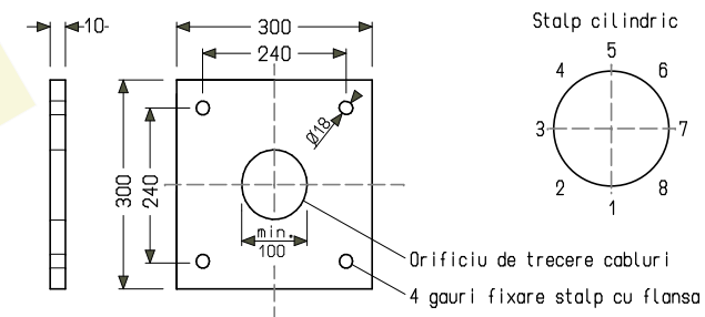
Detailu B - Flansa de prindere
