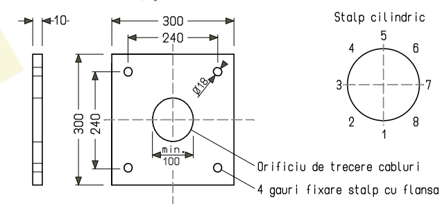
Detaliu B - Flansa de prindere
