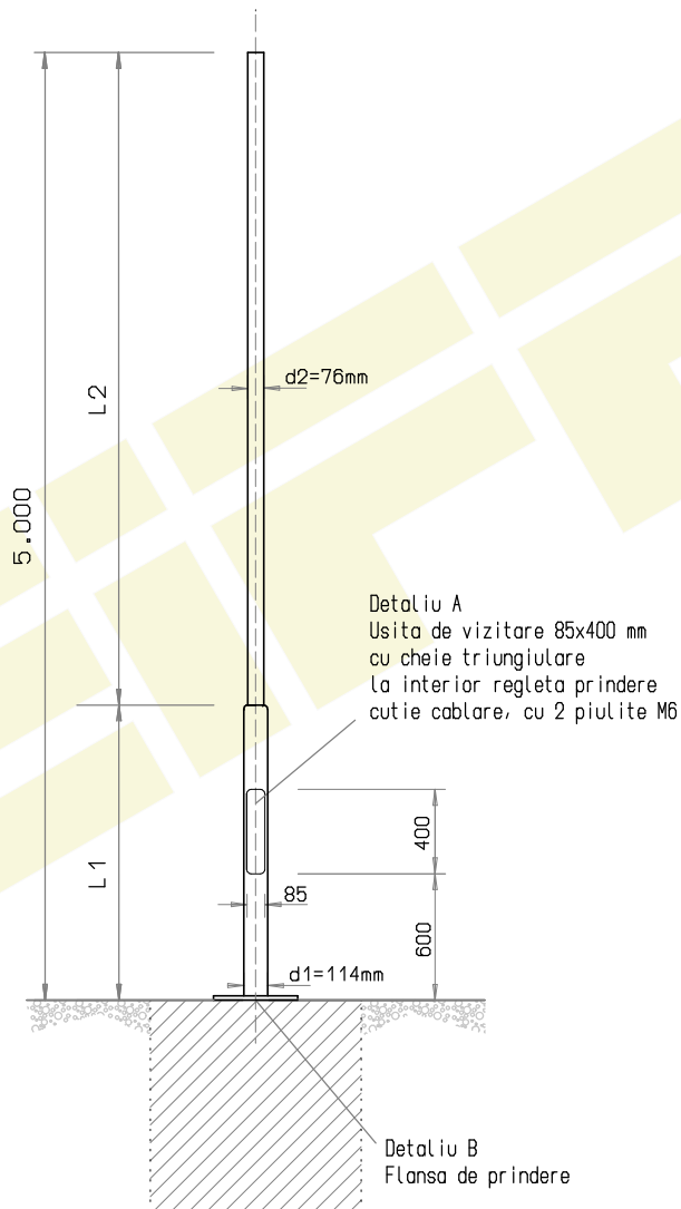
Detaliu B - Flansa de prindere
