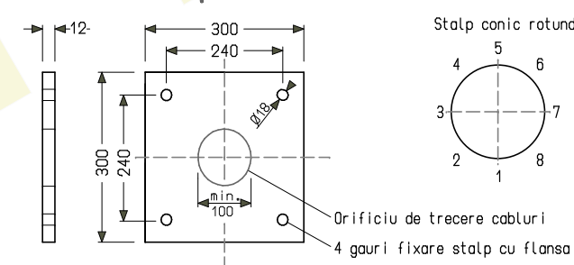
Vedere in sectiune
