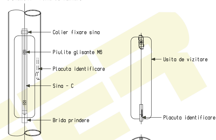
Detaliu A - Usita de vizitare
