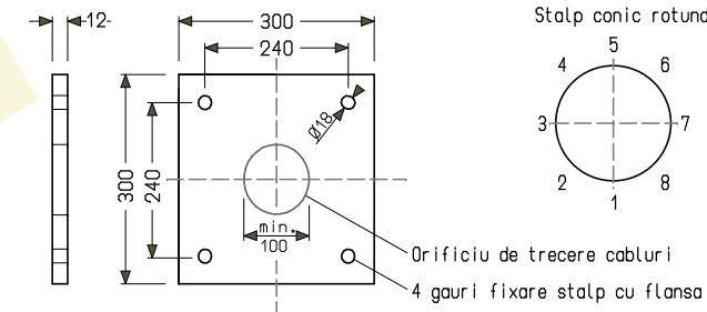
Detaliu B - Flansa de prindere
