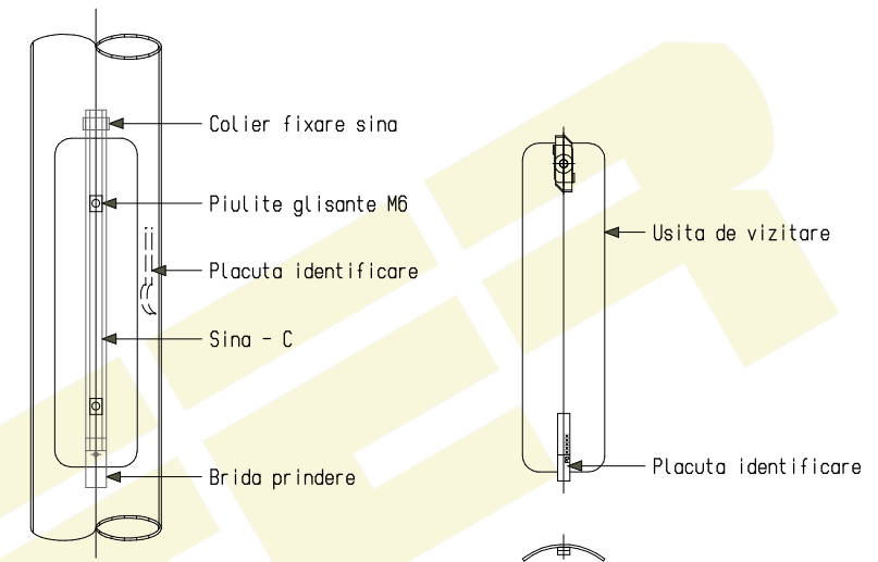
Detaliu A - Usita de vizitare
