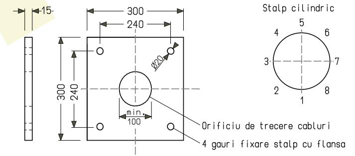
Detaliu B - Flansa de prindere
