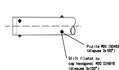
Detaliu D
